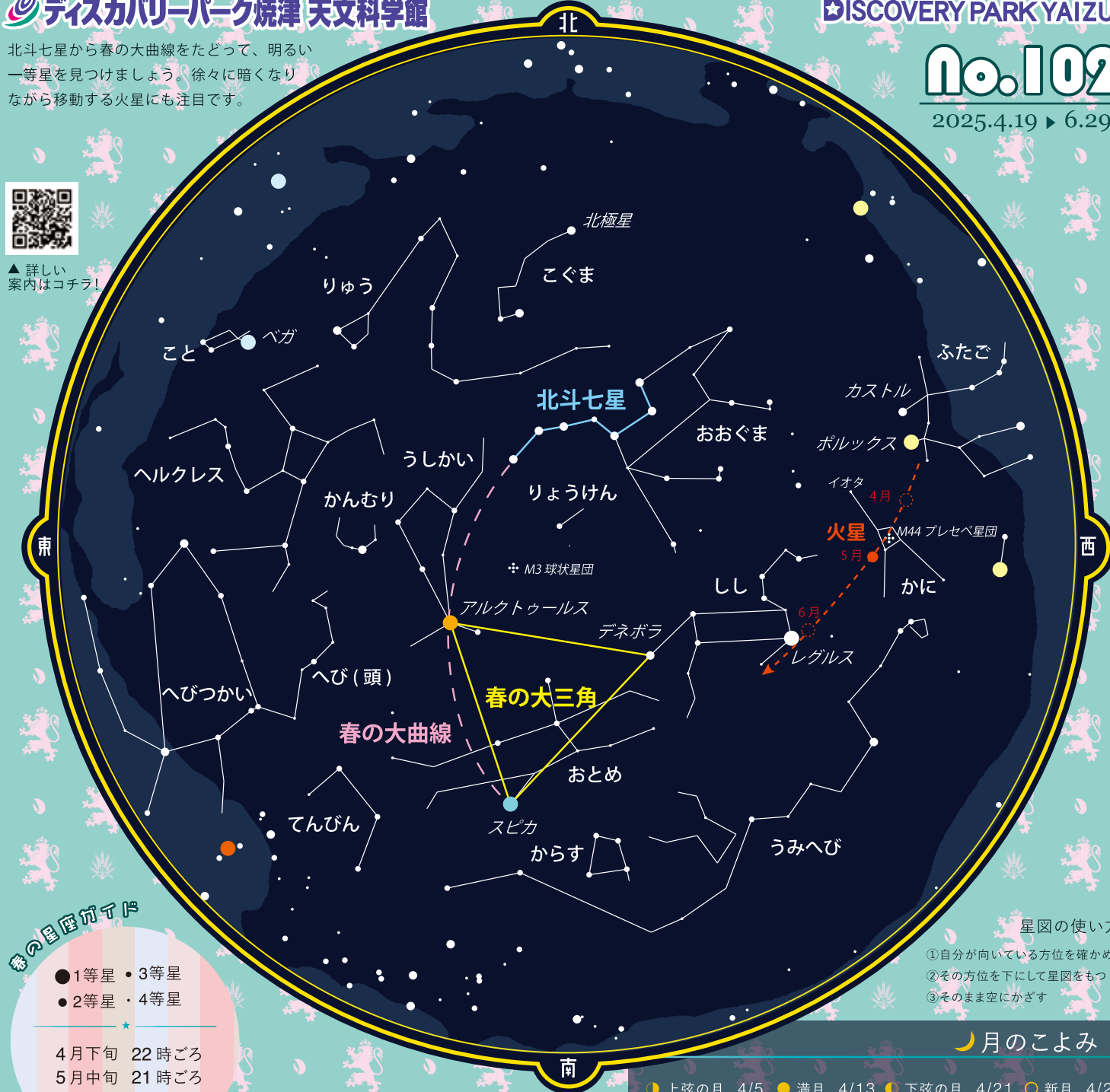
かに座イオタ星 (二重星)
