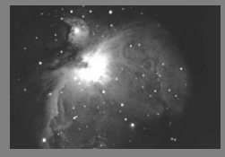
オリオン大星雲 : 12月～3月
